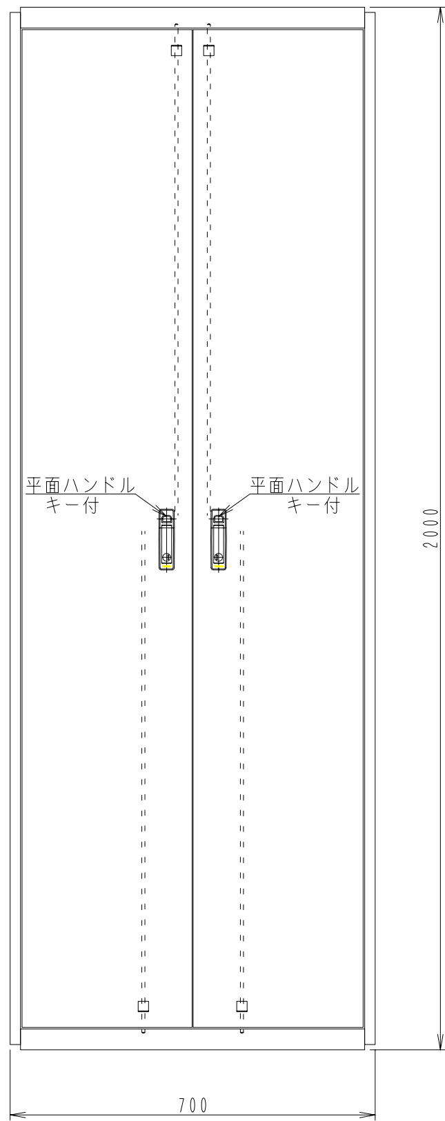
正面図
